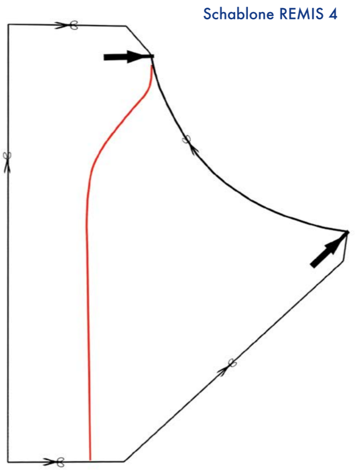
Einbau bei linker Tür / Jig for left door / gabarit de coupe pour la porte à gauche / sjabloon voor de deur links
